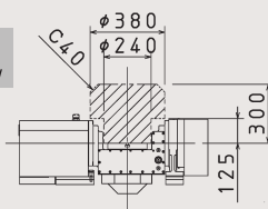
正面図 Front view
