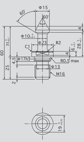
プルスタッド Pull stud MAS P40T-II
