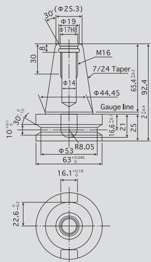
工具シャンク Tool shark MAS BT40
