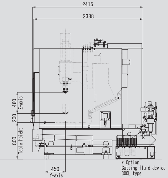
右側画面 Right view
