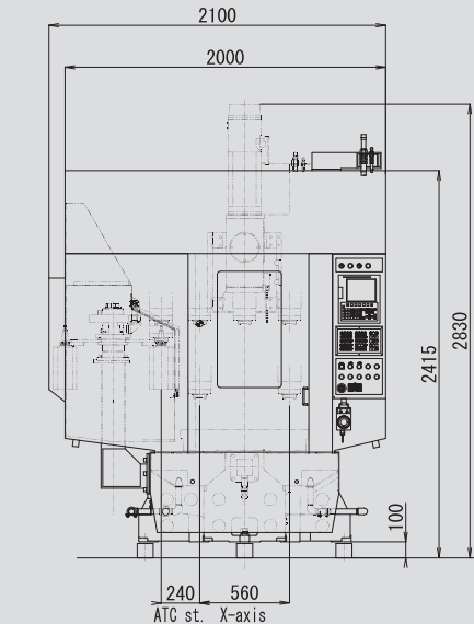
正面図 Front view
