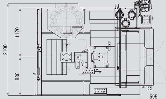
上画面 Top view
